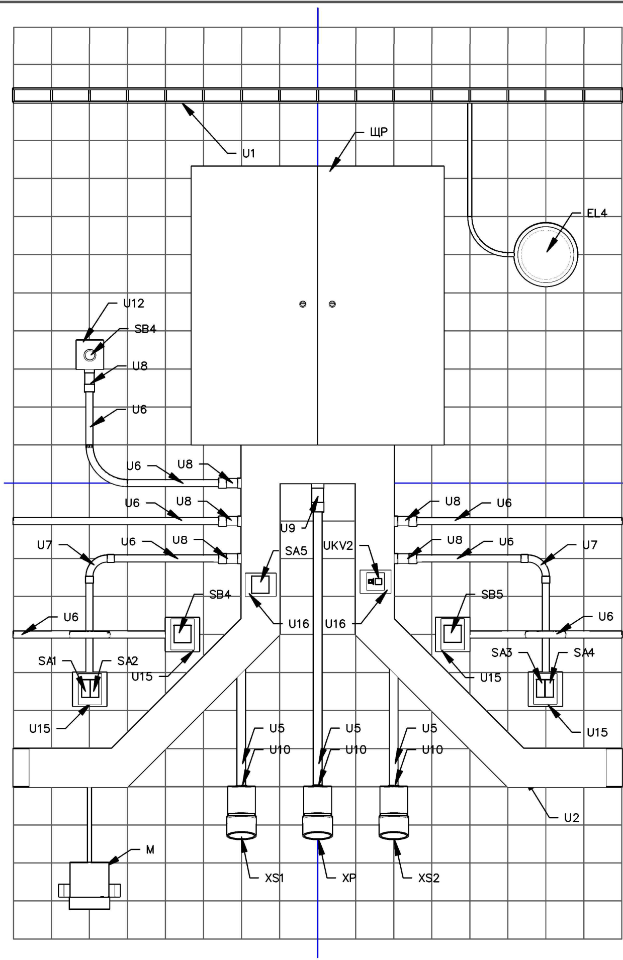
Монтажная схема вид "Б"
